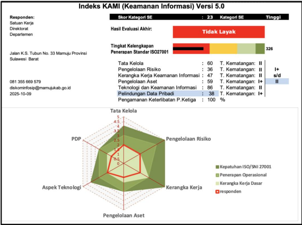
Gambar 4.8 Laporan Assessment Indeks Keamanan Informas (IKAMI) Versi 5.0 Pemerintah Kabupaten Mamuju Tahun 2025
